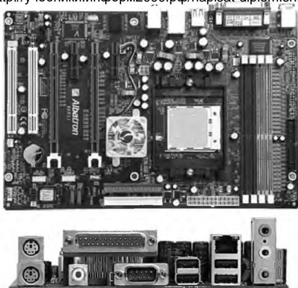
Рис. 4.5. Материнская плата
