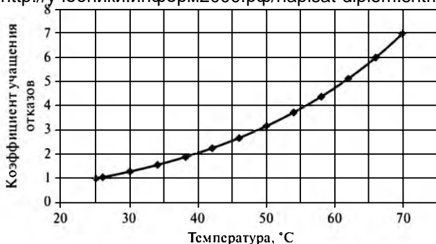
Рис. 4.13. Зависимость учащения отказов от повышения температуры винчестера (по данным Seagate Technology)
